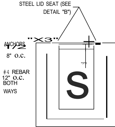
SECTION D-D
